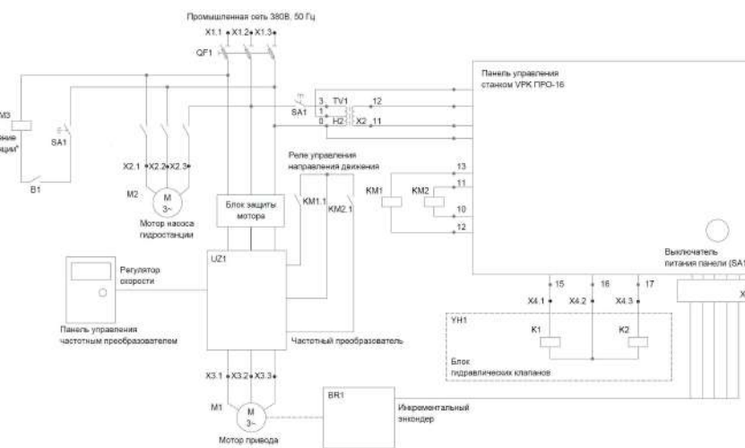
Рис. 4. Принципиальная электрическая схема станка
