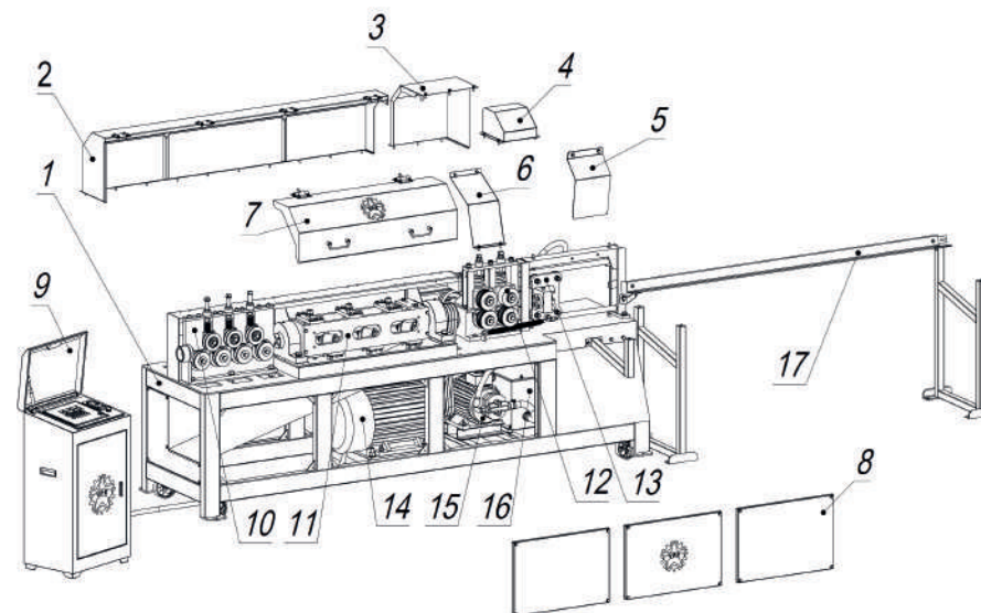
Рис. 1. Схема устройства правильно-отрезного станка ВКР ПРО-16:
